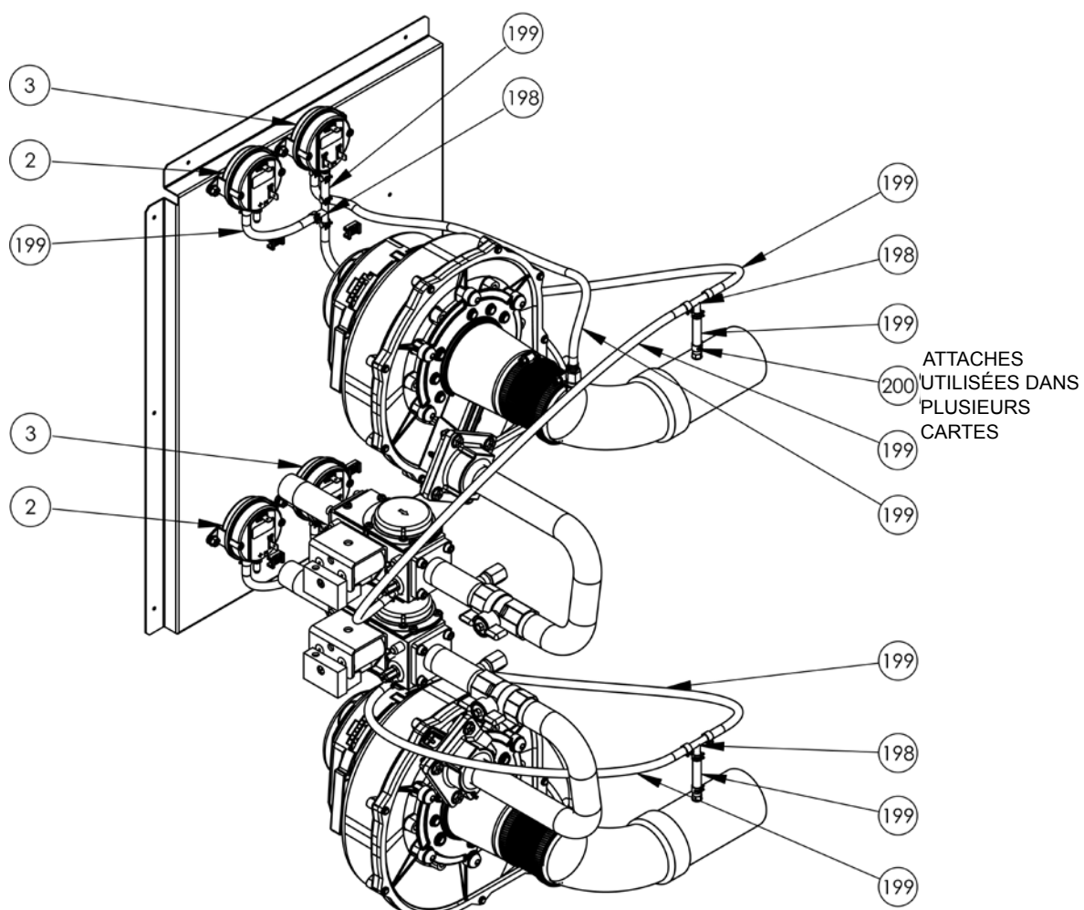
Figure 52. Détails du brûleur
