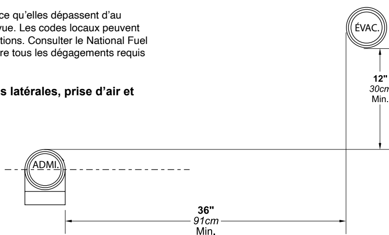
Figure 8. Distance minimale du conduit d'évacuation des gaz de combustion
