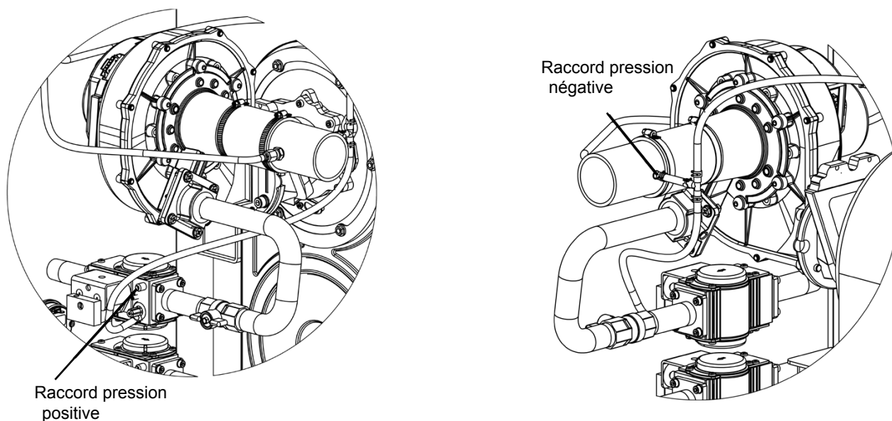
Figure 41. Raccords pour manomètre, NT 1000 et NT 1200
