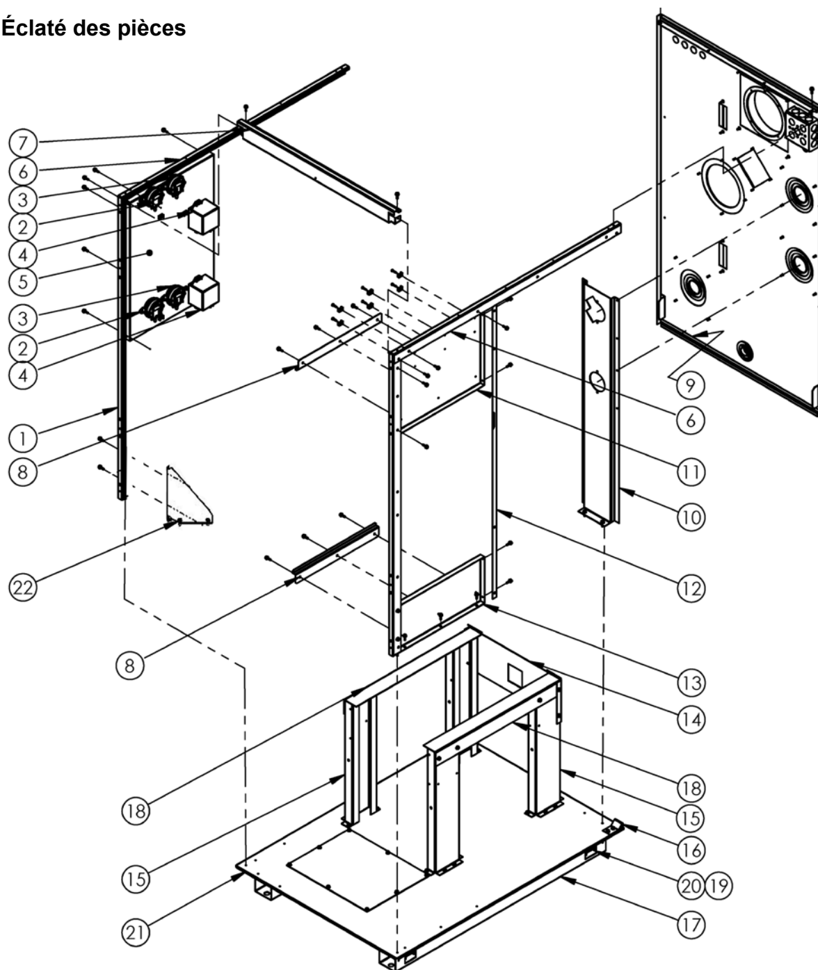
Figure 46. Châssis – NT1000 et NT1200
