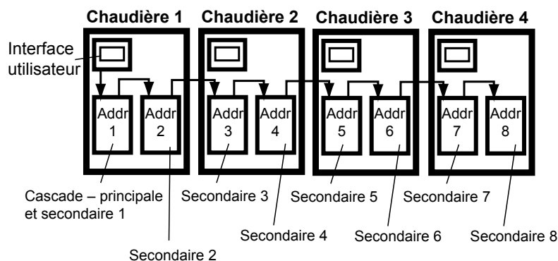
Figure 30. Mise en cascade dans un système à plusieurs chaudières
