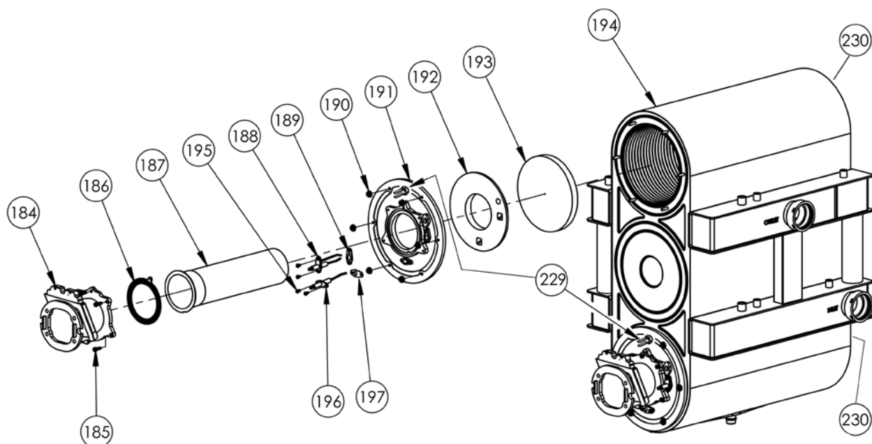
Figure 51. Composants de l'échangeur thermique
