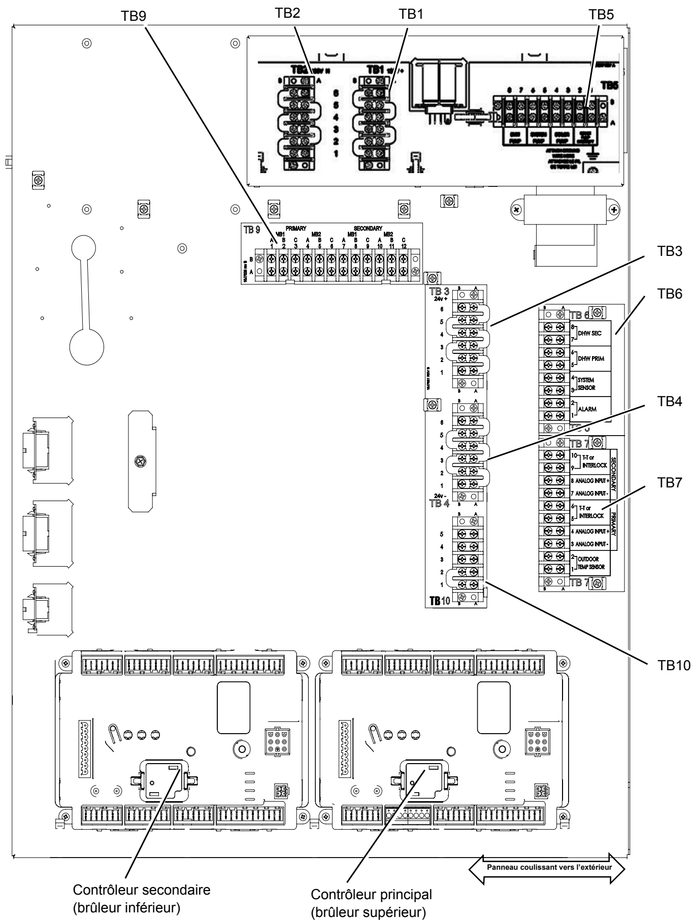
Figure 17. Schéma de la carte électronique
