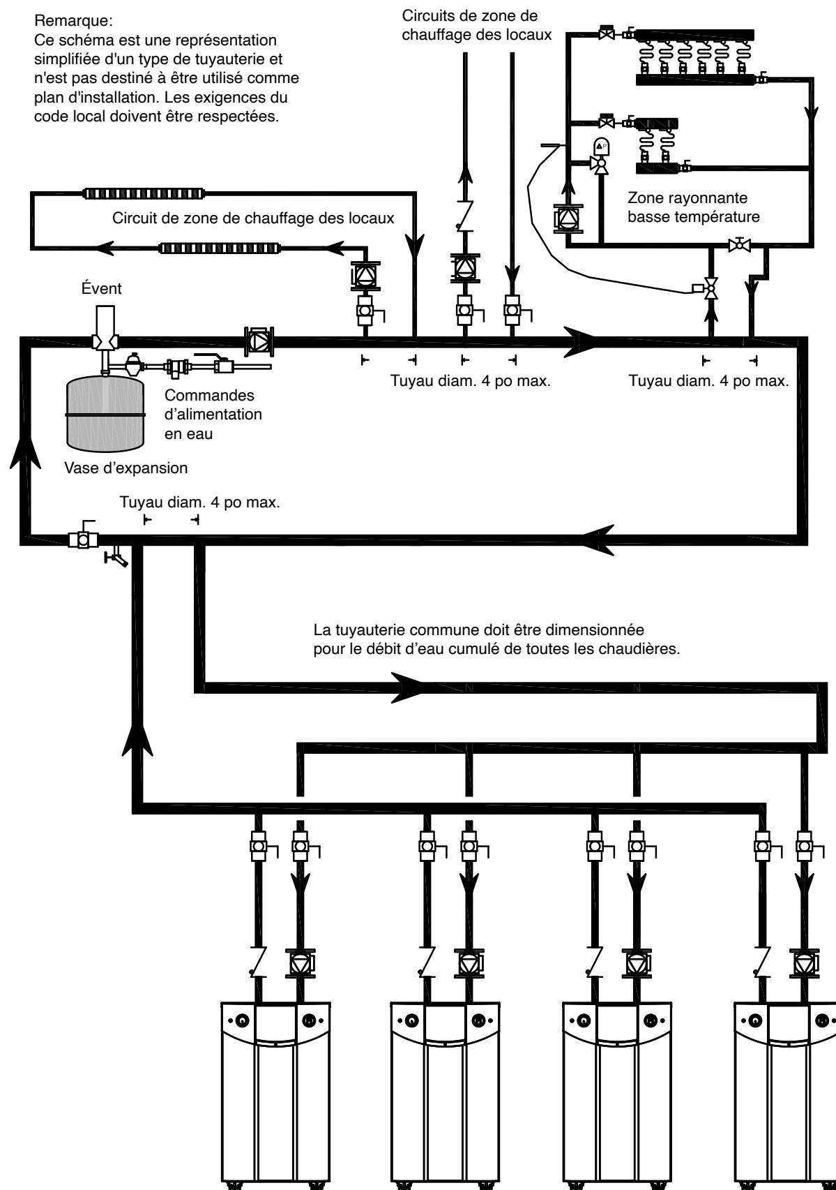
Figure 12. Tuyauterie chauffage – plusieurs chaudières, plusieurs zones de températures, à retour inversé Zonage avec circulateurs
