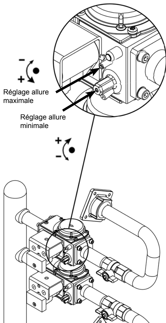
Figure 40. Réglages des allures minimale et maximale sur la vanne de gaz – NT 1000 et NT 1200
