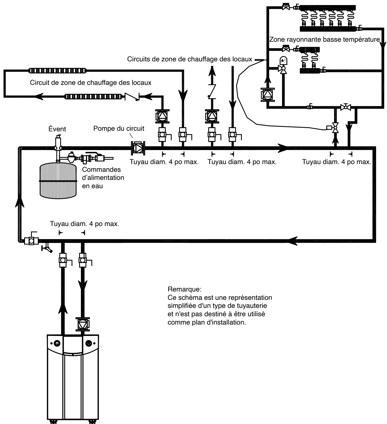
Figure 9. Tuyauterie chauffage – une seule chaudière, plusieurs zones de températures. Zonage avec circulateurs
