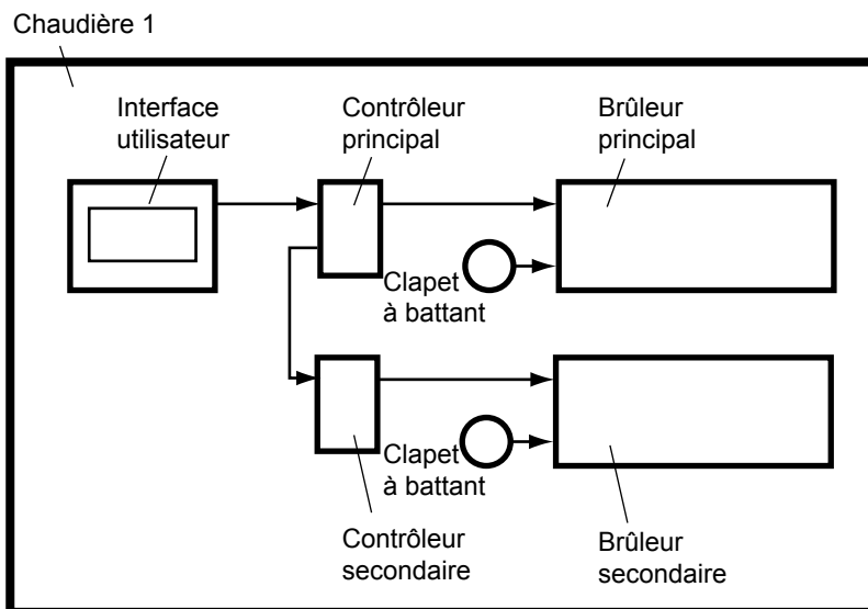
Figure 45. Configuration des clapets à battant
