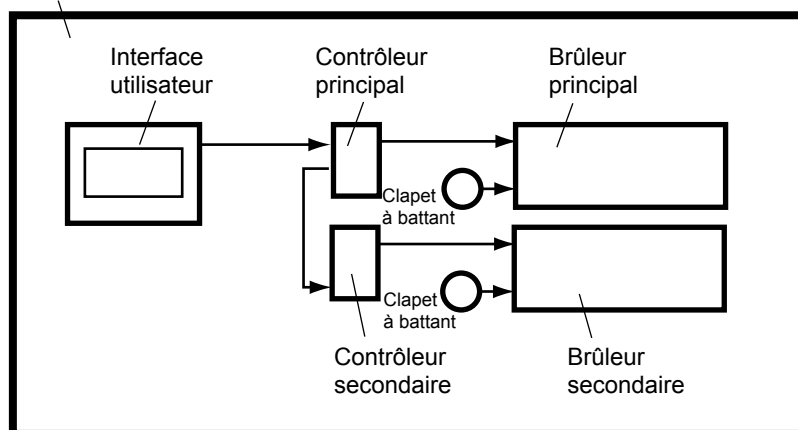
Figure 37. Configuration des clapets à battant
