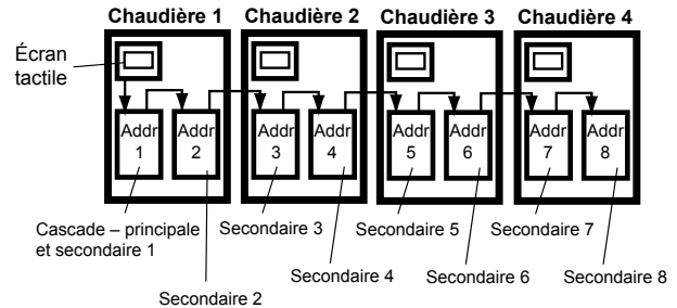
Figure 23. Mise en cascade dans un système à plusieurs chaudières
