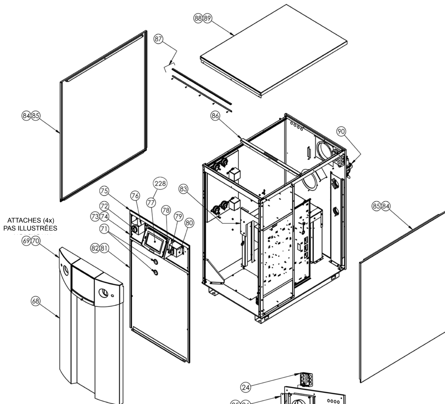
Figure 47. Panneaux et capots avant
