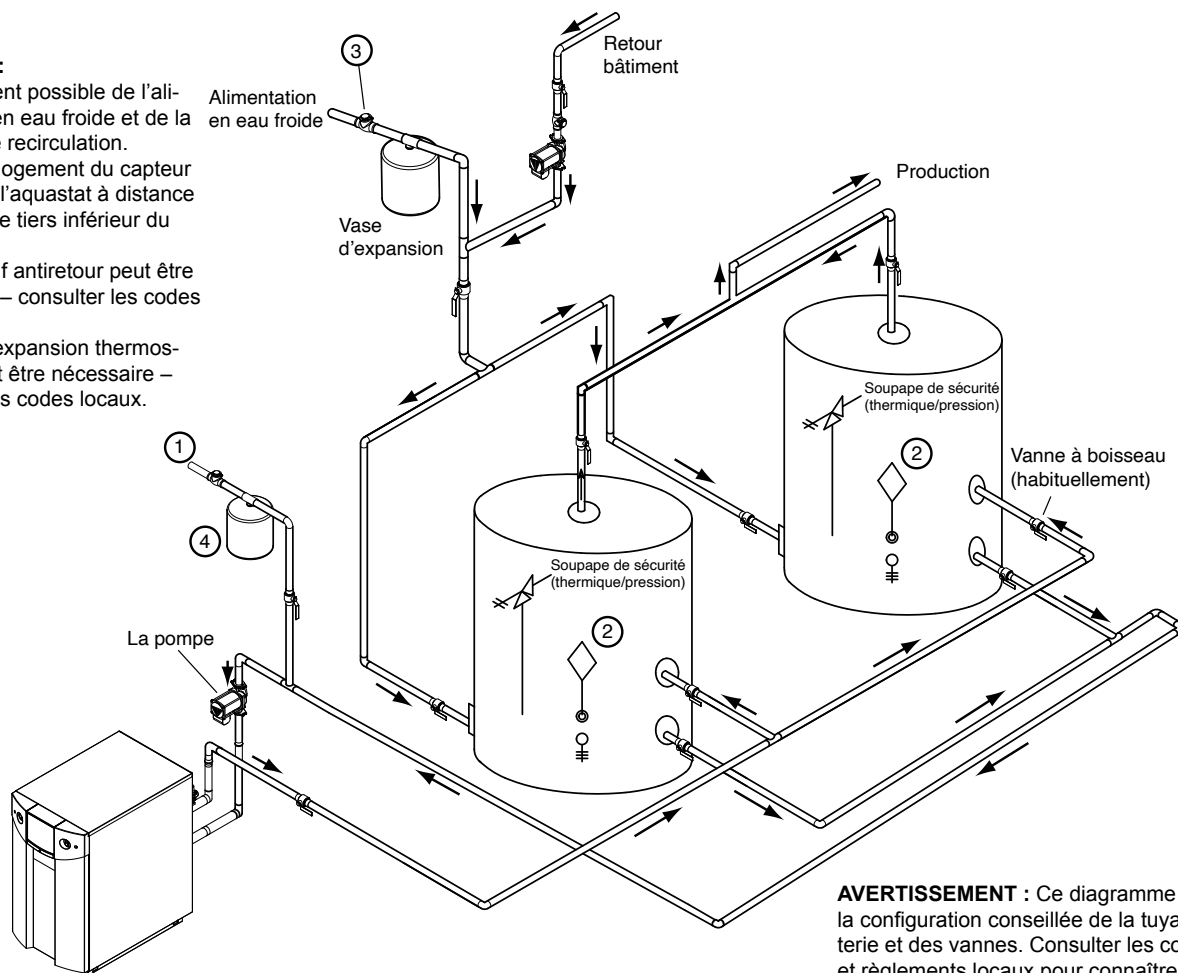
Figure 15. Tuyauterie ECS – un chauffe-eau, deux réservoirs verticaux
