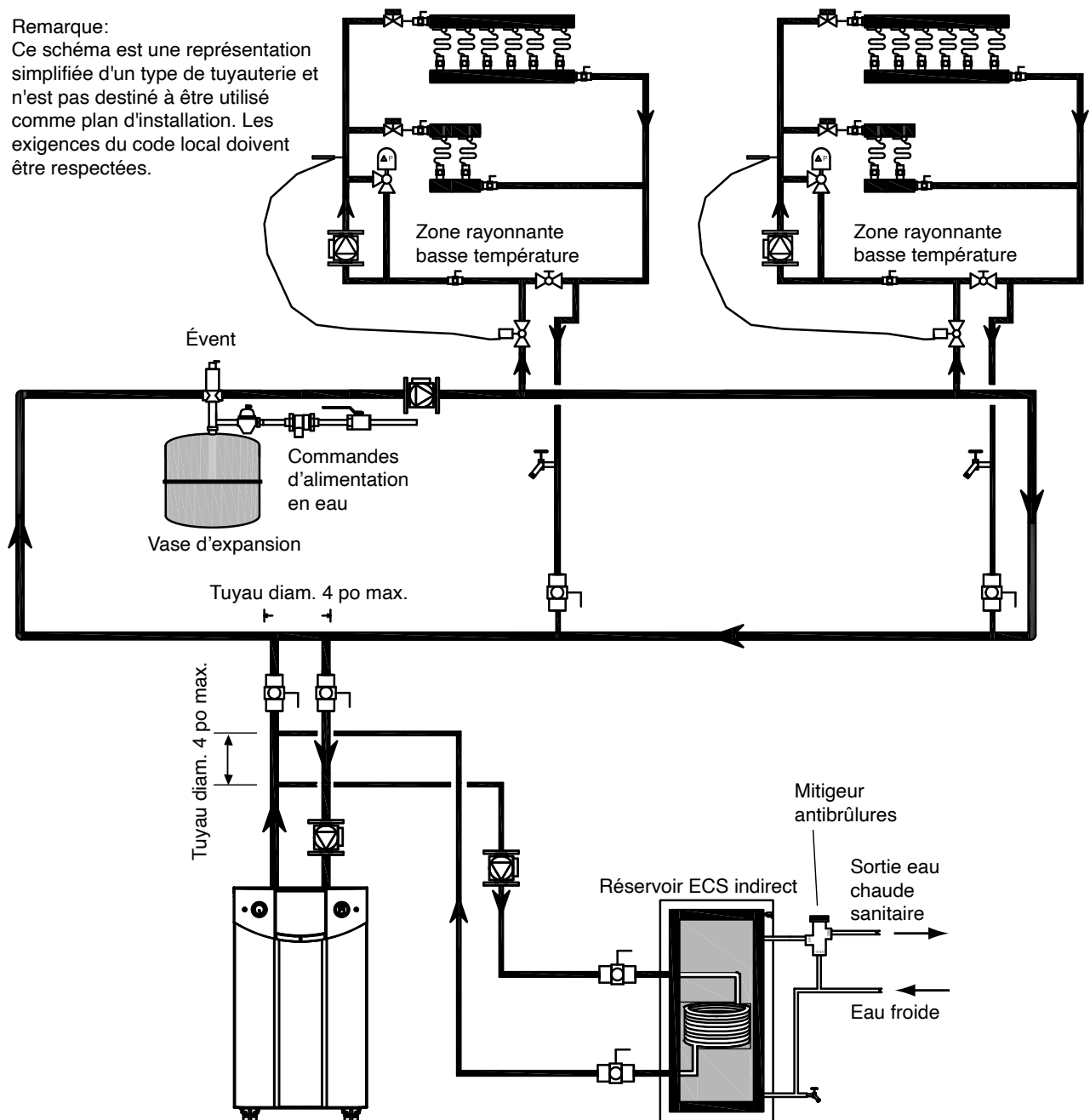
Figure 11. Tuyauterie chauffage – une seule chaudière avec des zones basse température et ballon eau chaude sanitaire indirecte
