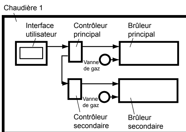
Figure 29. Mise en cascade dans un système à une chaudière
