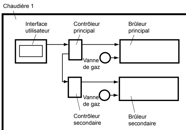
Figure 39. Brûleurs principal et secondaire dans une chaudière
