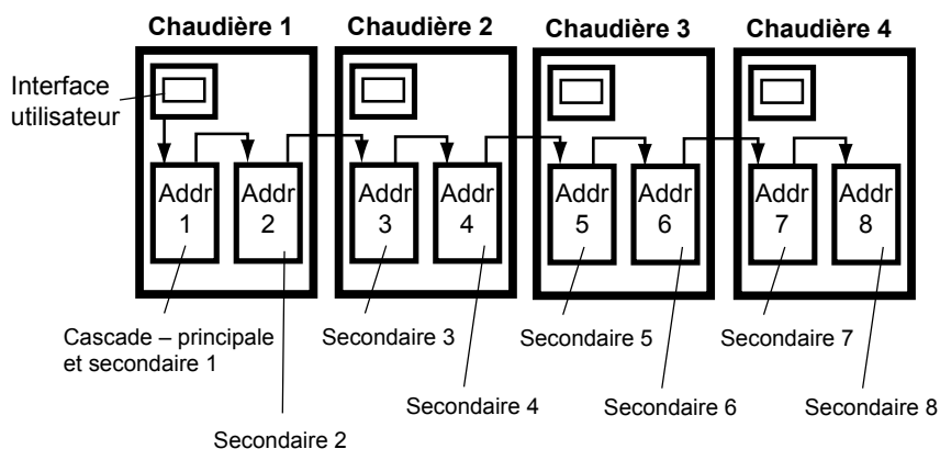
Figure 44. Mise en cascade dans un système à plusieurs chaudières
