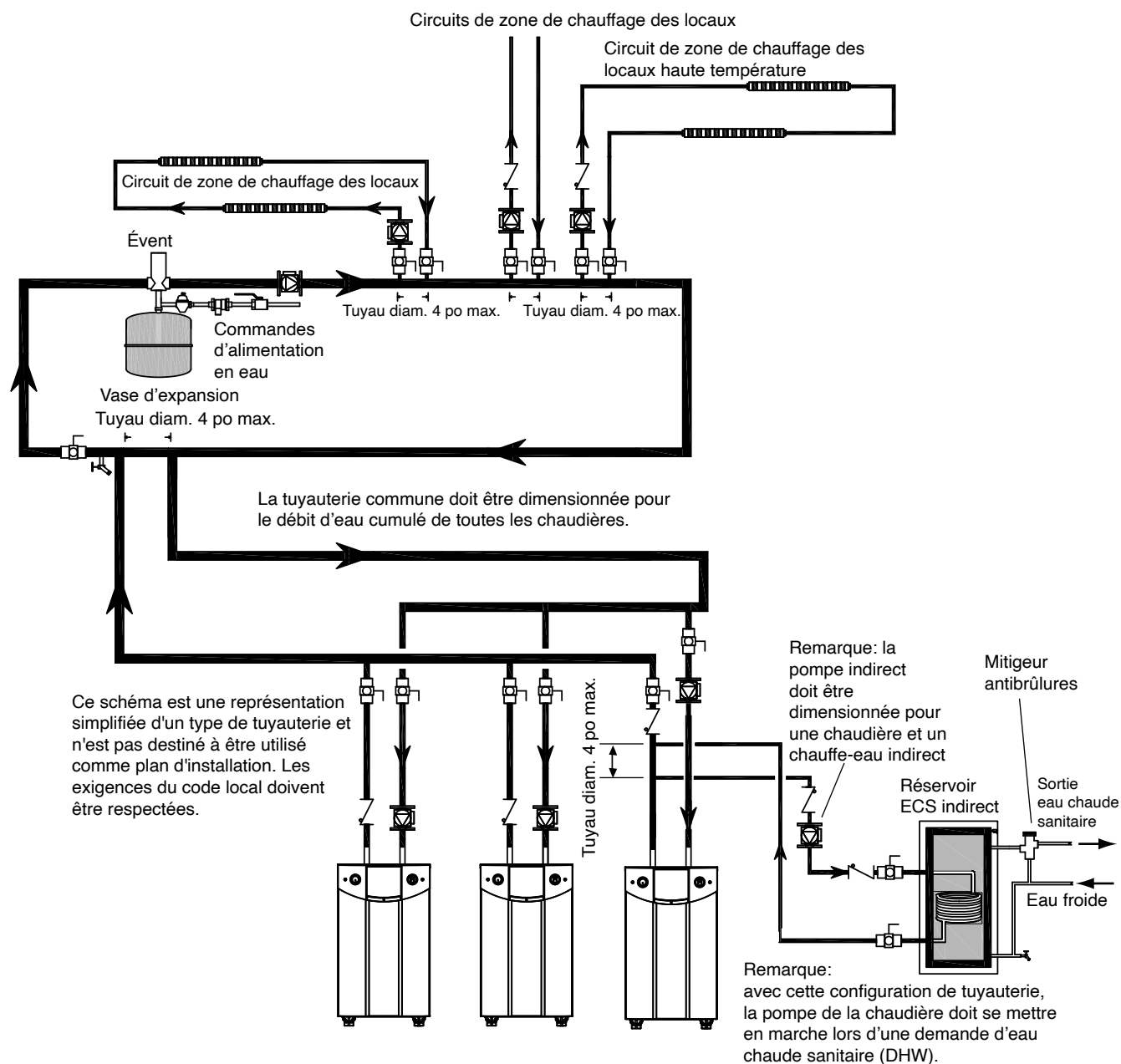
Figure 13. Tuyauterie chauffage – plusieurs chaudières, ballon eau chaude sanitaire (indirect) raccordé à une seule chaudière
