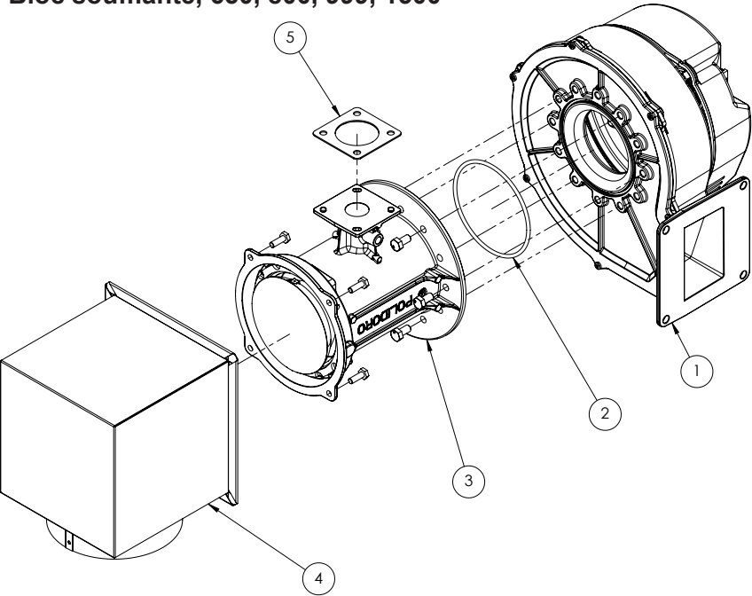
Bloc soufflante, 650, 800, 999, 1500
