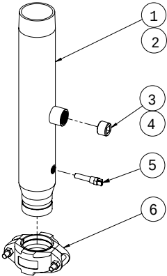
Tuyau d'entrée, toutes les dimensions
