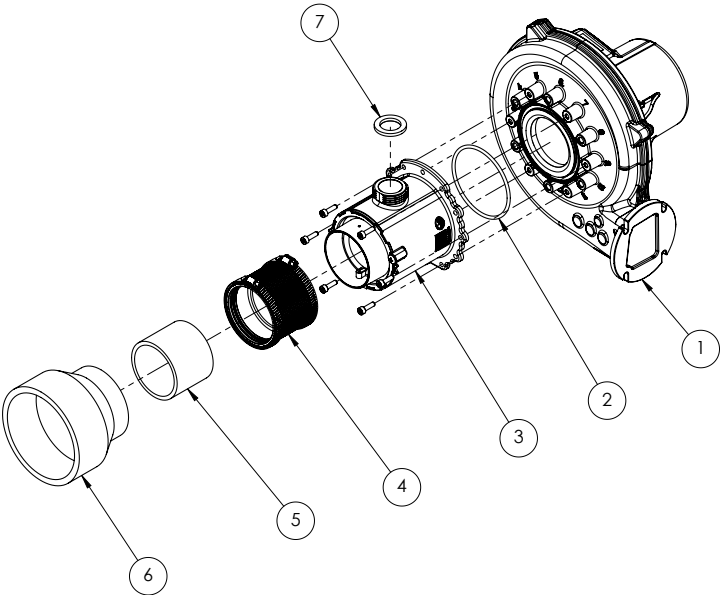
Bloc soufflante, 399 et 500
