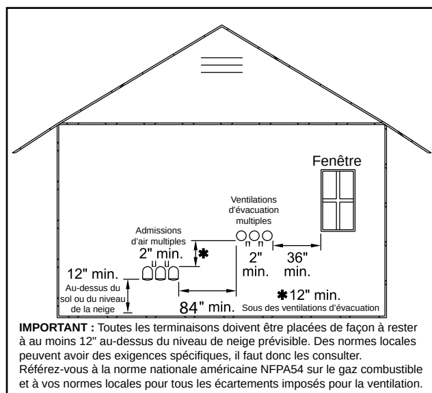
Figure 5. Terminaisons multiples d'air de combustion, ventilation sur murs latéraux
