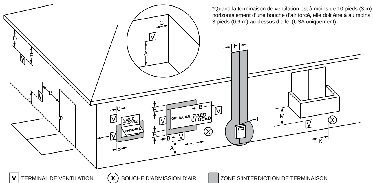
Figure 3. Air de combustion et ventilation au travers d'un mur latéral
