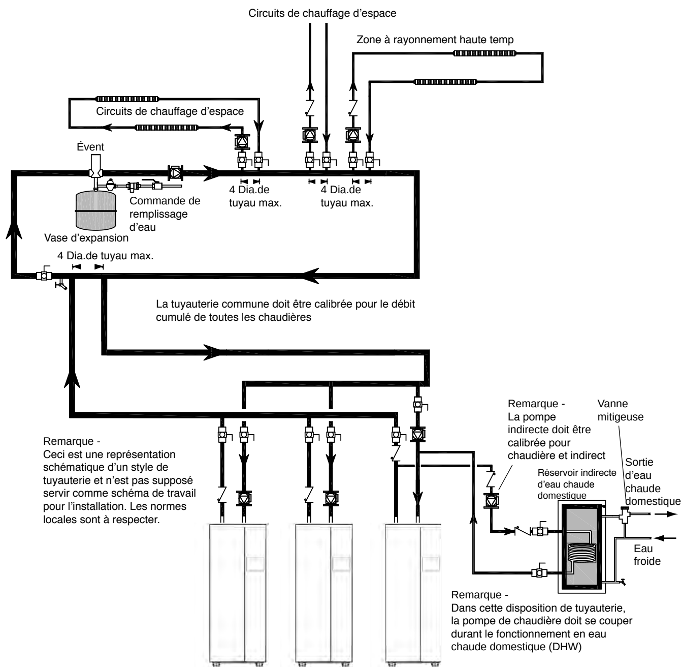
Figure 10. Tuyauterie hydronique — Plusieurs chaudières, DHW indirect coupé d'une chaudière
