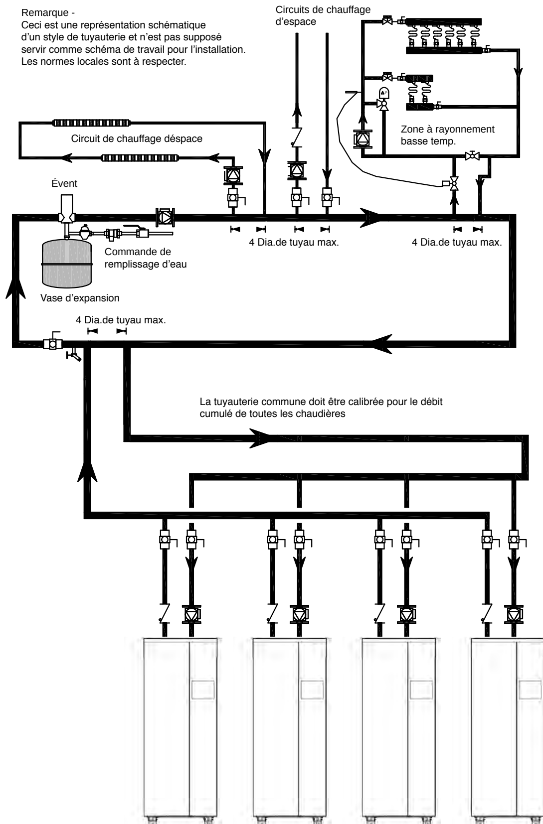
Figure 9. Tuyauterie hydronique — Plusieurs chaudières, plusieurs zones de température, retour inversé Zonage avec des circulateurs
