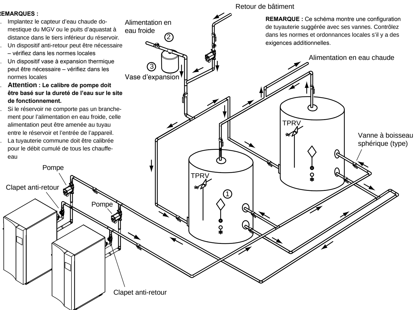
Figure 13. Tuyauterie d'eau chaude domestique (DHW) – Deux chauffe-eau, deux réservoirs verticaux
