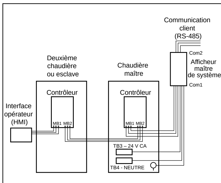
Figure 28. Connexions de BAS vers un système maître/esclave(s)
