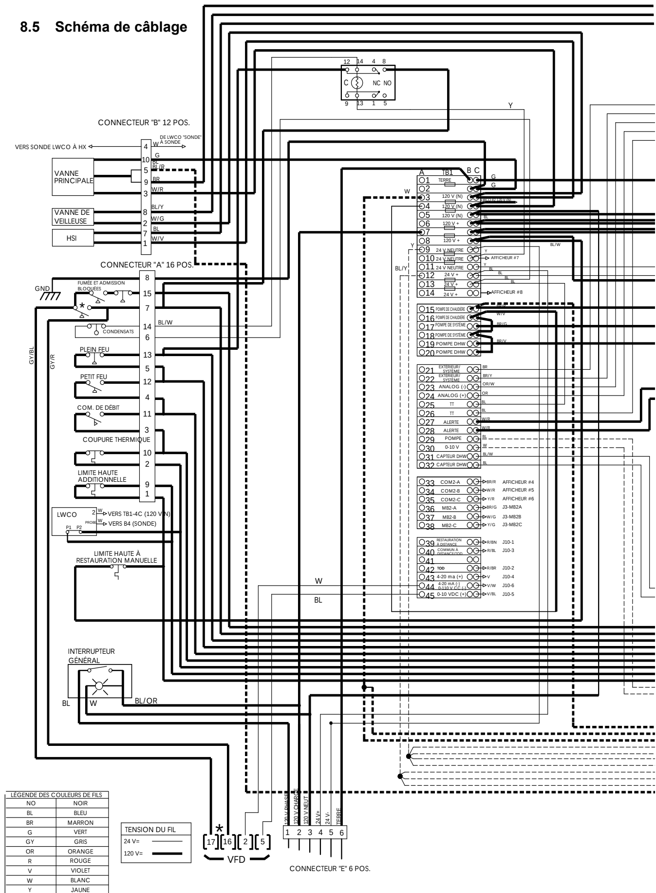
Figure 15. Schéma de câblage, tous les appareils
