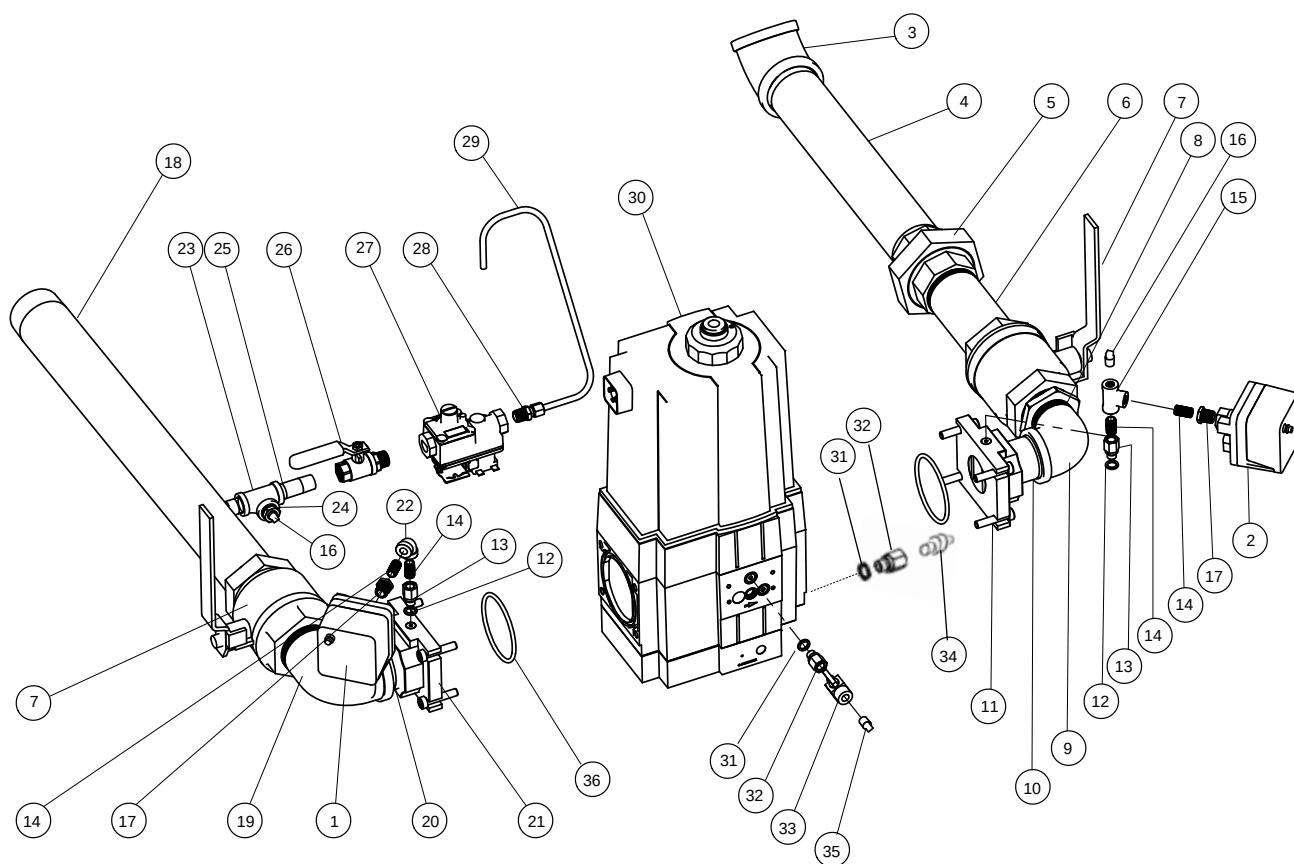
Ensemble de circuit de gaz (Modèle 3500 et 4000)
