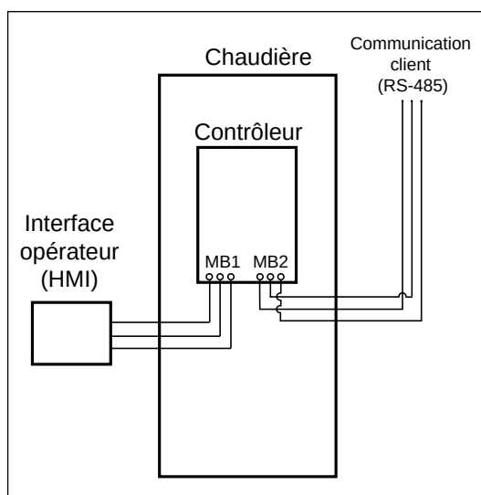
Figure 29. Connexions de BAS vers une chaudière unique
