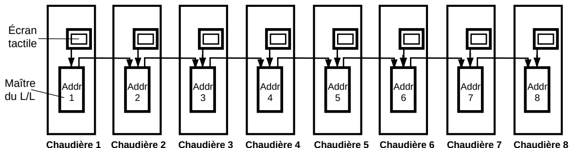
Figure 26. Fonctionnement en maître/esclave (L/L) avec huit chaudières.
