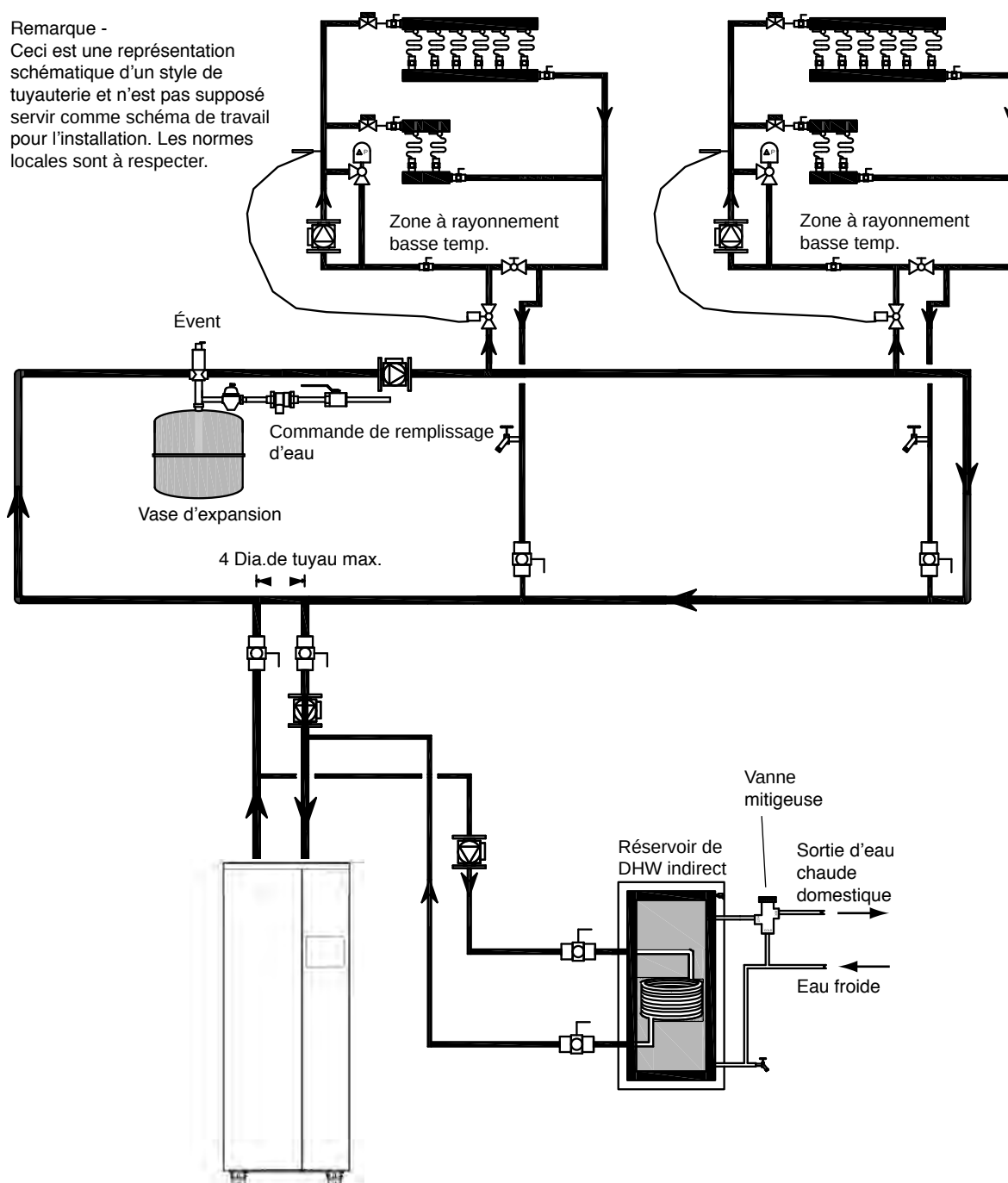
Figure 8. Tuyauterie hydronique — Chaudière unique avec zones à basse température et réservoir d'eau chaude domestique (DHW) indirect Réservoir indirect en sortie de chaudière
