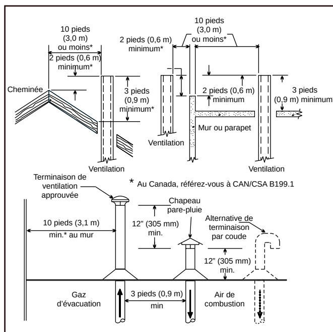
Figure 6. Air de combustion et ventilation au travers du toit
