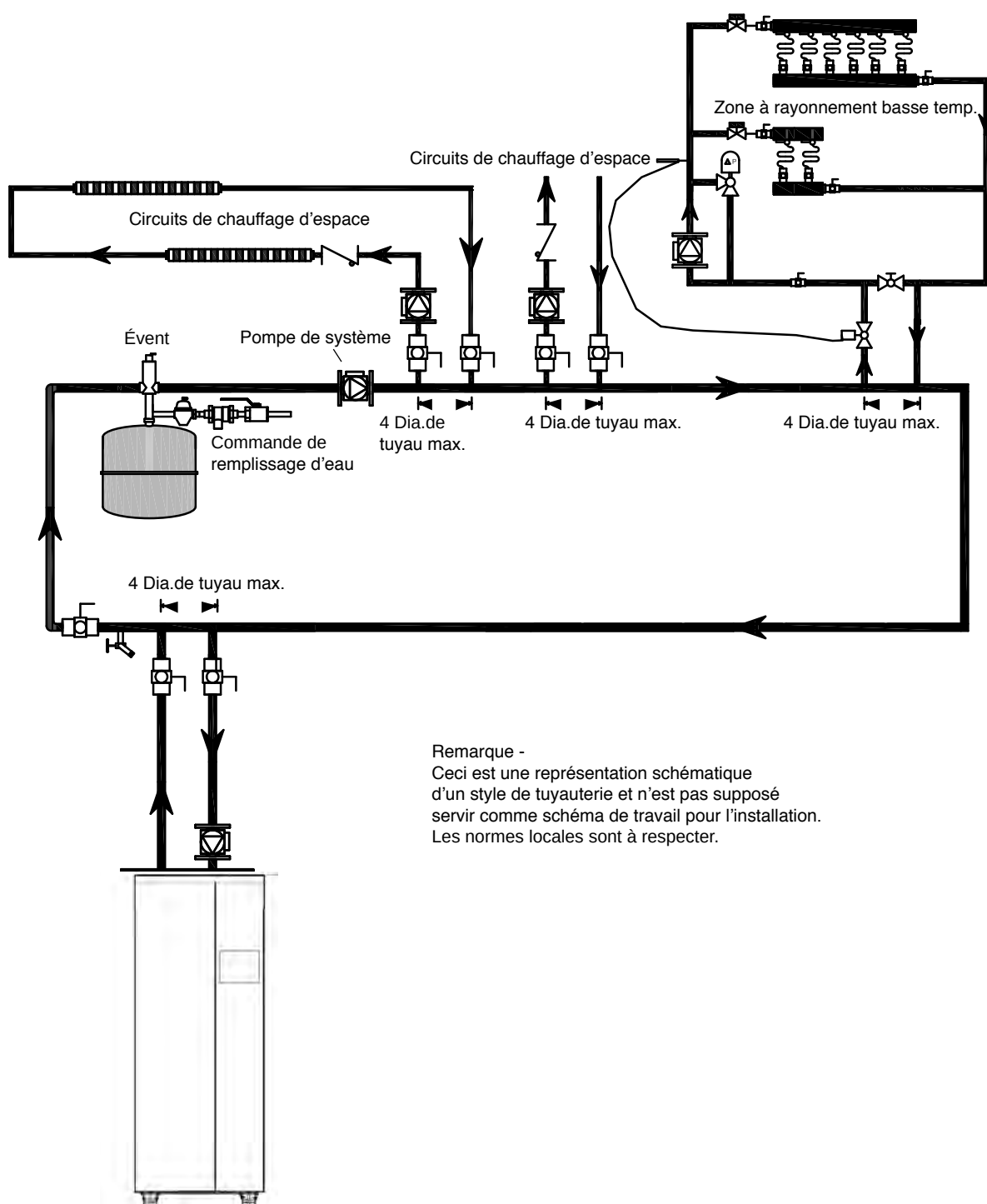
Figure 7. Tuyauterie hydronique — Chaudière unique, plusieurs zones de température Zonage avec des circulateurs
