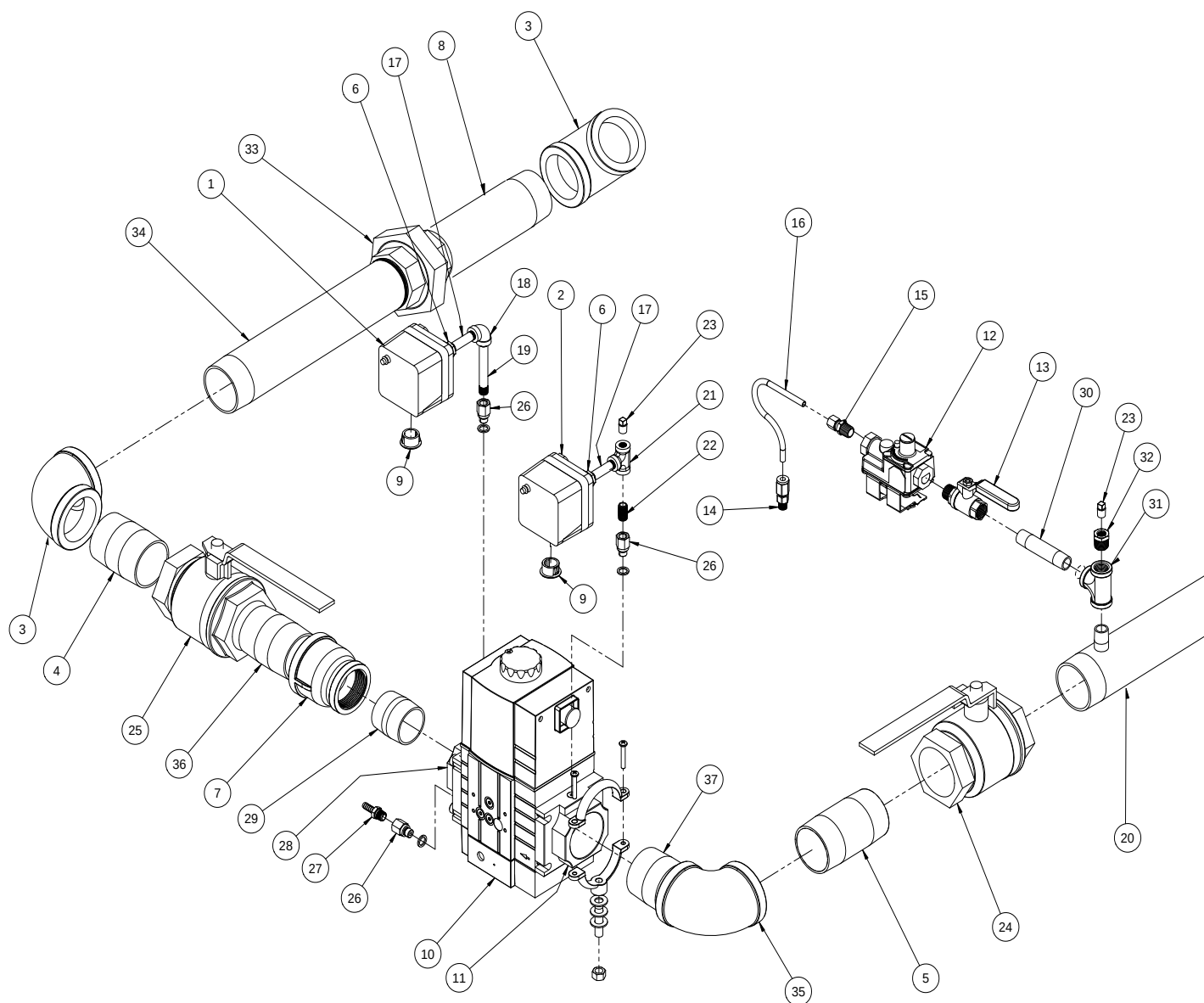
Ensemble de circuit de gaz (Modèles 2000, 2500 et 3000)
