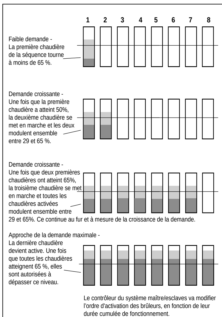
Figure 27. Fonctionnement Maître/Esclave avec 3 chaudières ou plus
